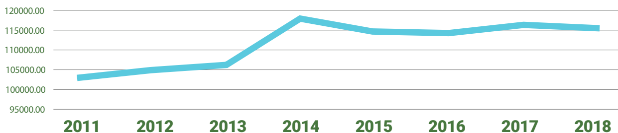
54-nji surat. 2011–2018-nji ýyllarda göni parnik gazlarynyň emissiýasy, Gg (CO 2 -ekw.)
